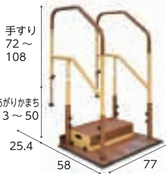
両手すり BZD-04WD(N)
