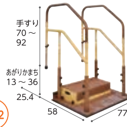
両手すり BZD-08WD(N)
